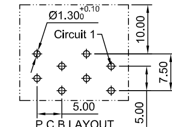
P.C.B LAYOUT -COMPONENT SIDE HDGC7921WRA-RH-XP-**-(-TH*)
