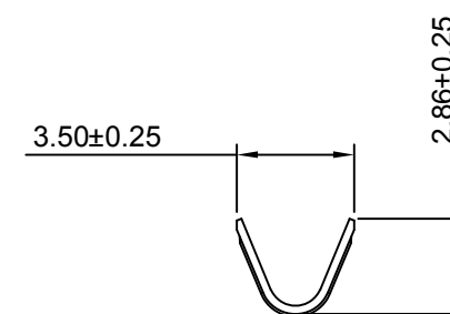
SEC:B-B
