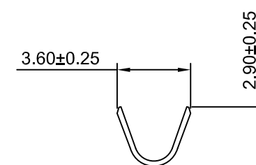
SEC:B-B
