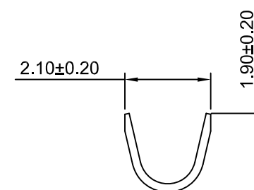
SEC:A-A
