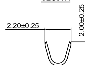
SEC:B-B
