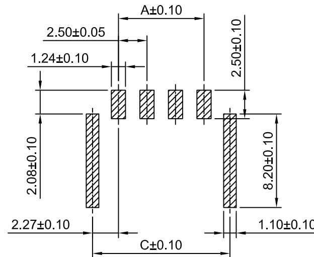
P.C.B LAYOUT
