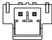
2x2P KEY B
