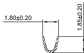
SEC:B-B
