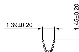
SEC:B-B
