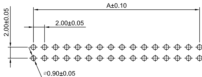
P.C.B LAYOUT
