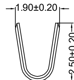
SEC:A-A
