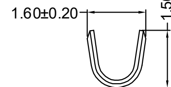
SEC:B-B
