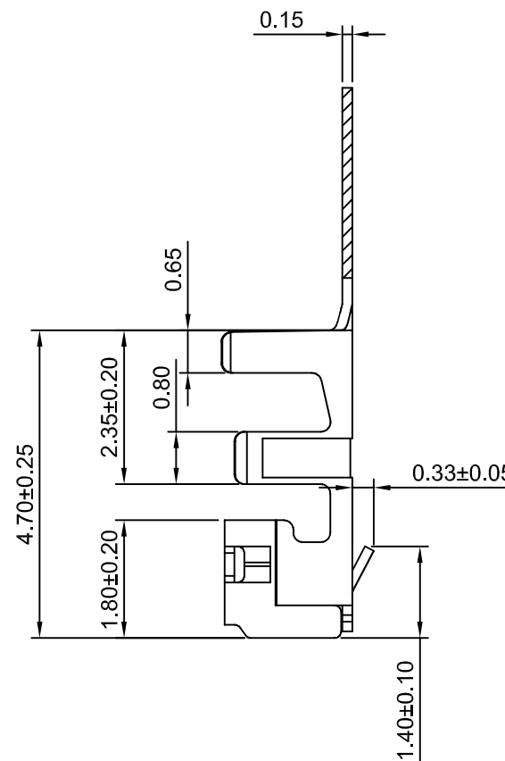
SEC: B-B
