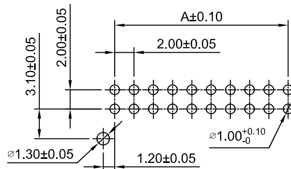
P.C.B LAYOUT
