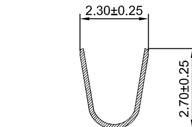
SEC:A-A
