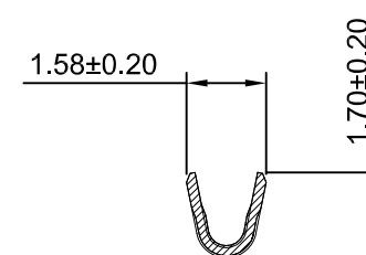
SEC: B-B
