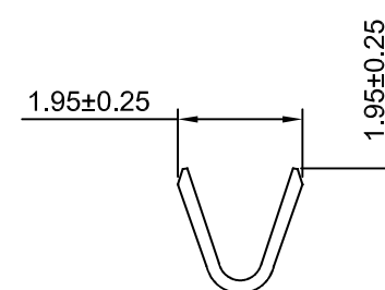
SEC:A-A
