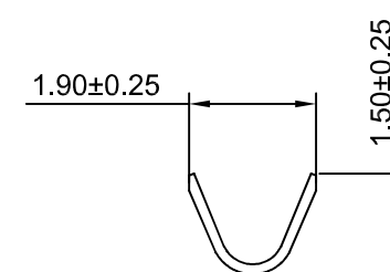
SEC:B-B
