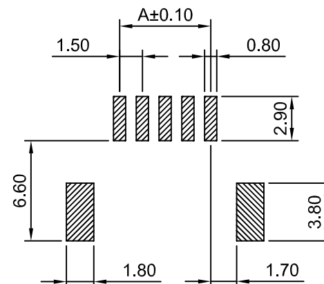
P.C.B LAYOUT
