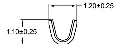
SEC:B-B
