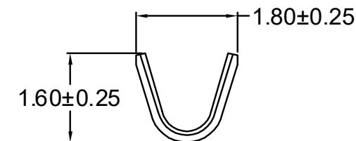
SEC:A-A
