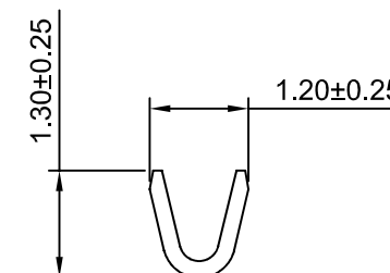
SEC:B-B
