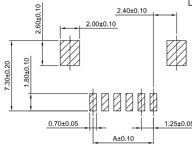
P.C.B. LAYOUT
