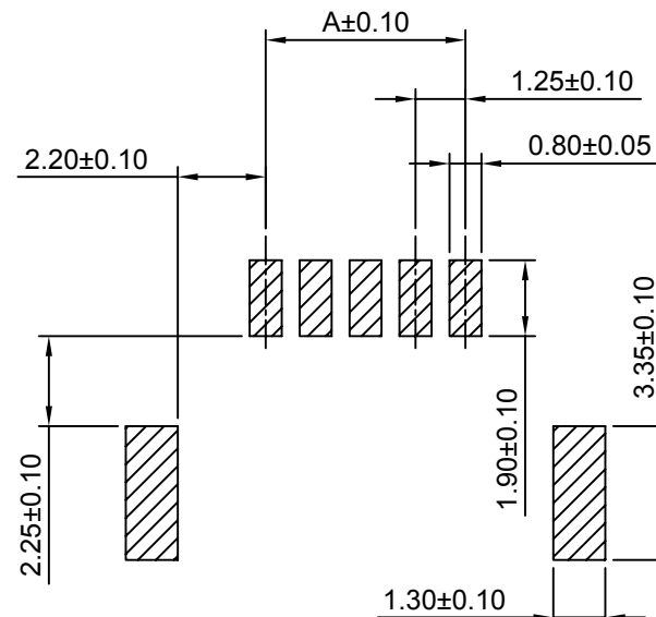
P.C.B. LAYOUT
