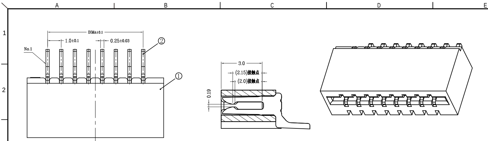
SECTION A-A
