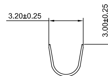
SEC:A-A
