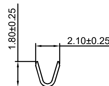
SEC:B-B
