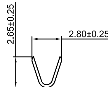
SEC:A-A
