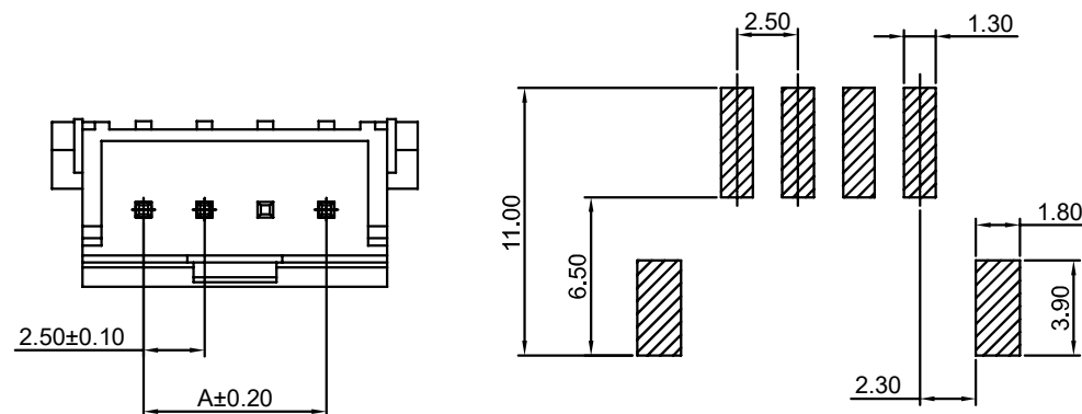
P.C.B LAYOUT
