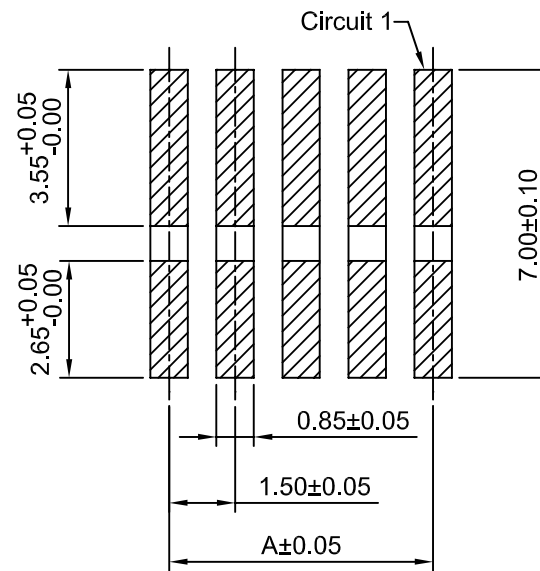
P.C.B LAYOUT
