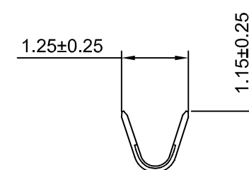
SEC:B-B
