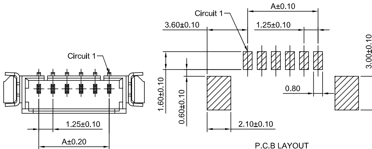
P.C.B LAYOUT
